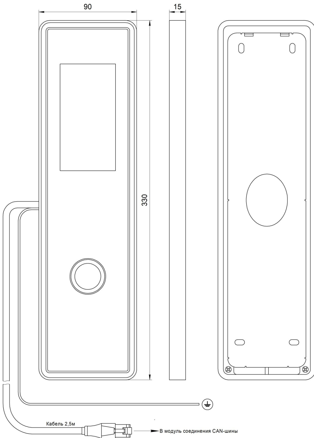
Рис.1 Внешний вид, габаритные и установочные размеры Вызывного поста ОБСИДИАН (жгут RJ45) НШЕК.468381.219
